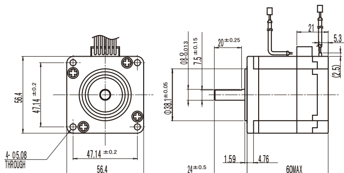
片軸 (S) タイプ
