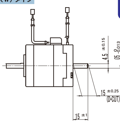
両軸 (W) タイプ
